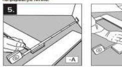
5. Отмерьте и нарежьте завершающие панели по размеру. Завершите первый ряд с помощью полученных панелей. Убедитесь, что вы оставили зазор не менее 8 мм от стены.
